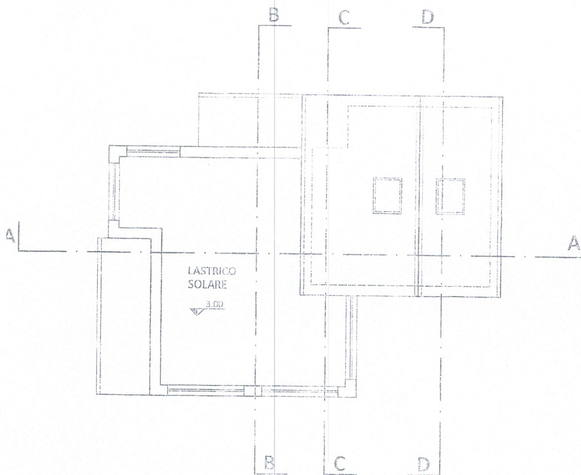
PIANTA COPERTURA
